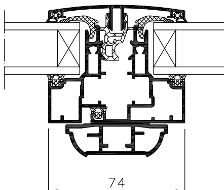
Battement centré extra réduit (option)
