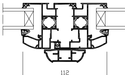
Frappe traditionnelle : design droit, parclores montants galbées (option)
