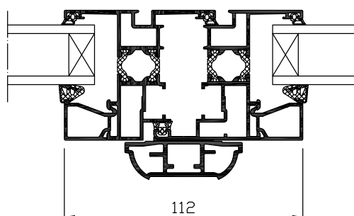
Battement centré de 112 mm
