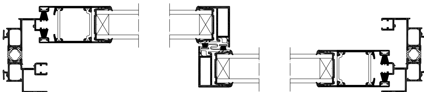
Coulissant : design droit, montant chicane extra réduit
