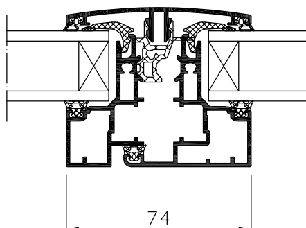
Battement extra réduit
