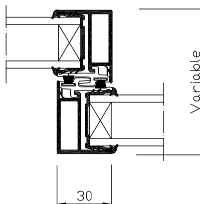
Coulissant : Montant chicane extra réduit : 30 mm
