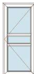
PE 2T 2 TRAVERSES HORIZ.
