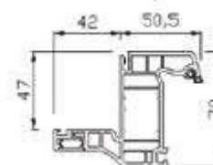
Réno cille de 42 mm compensée
