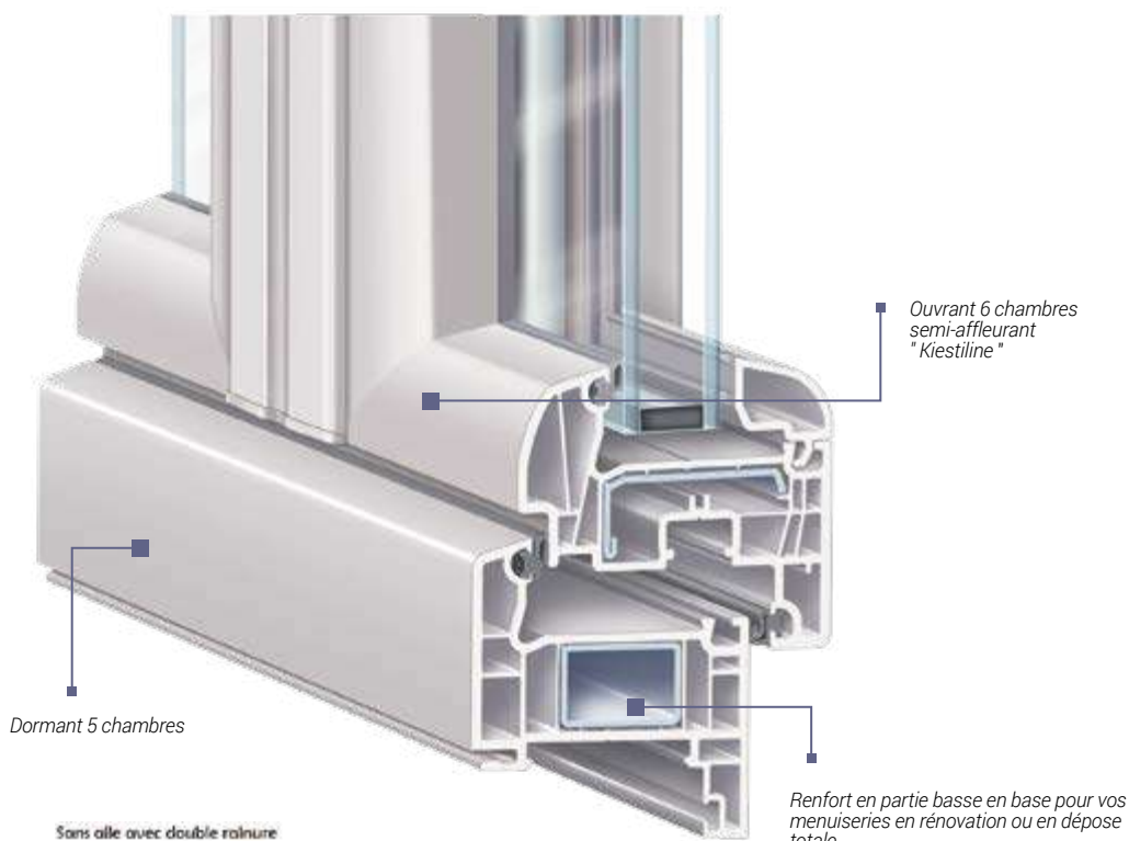
Sans aile avec double rainure
